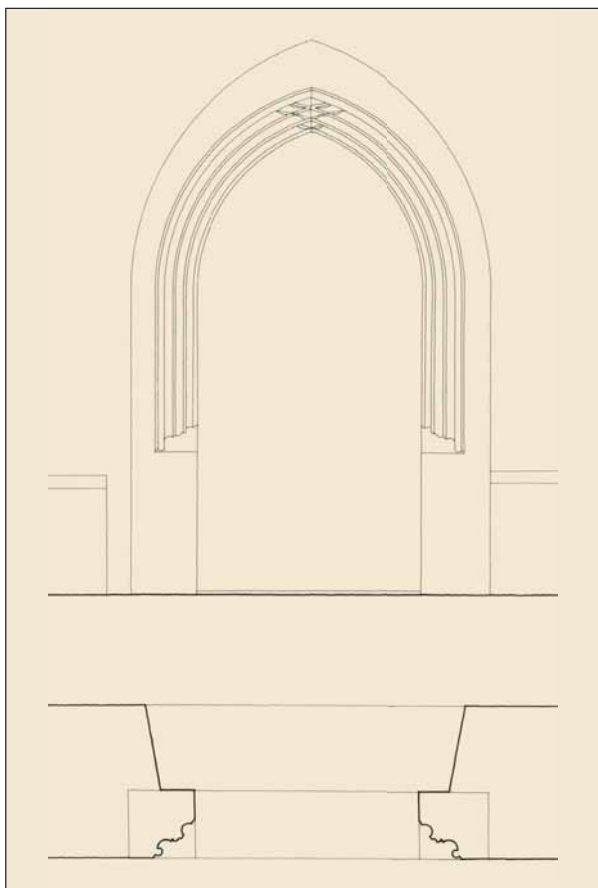
3. Releveul portalului vestic
