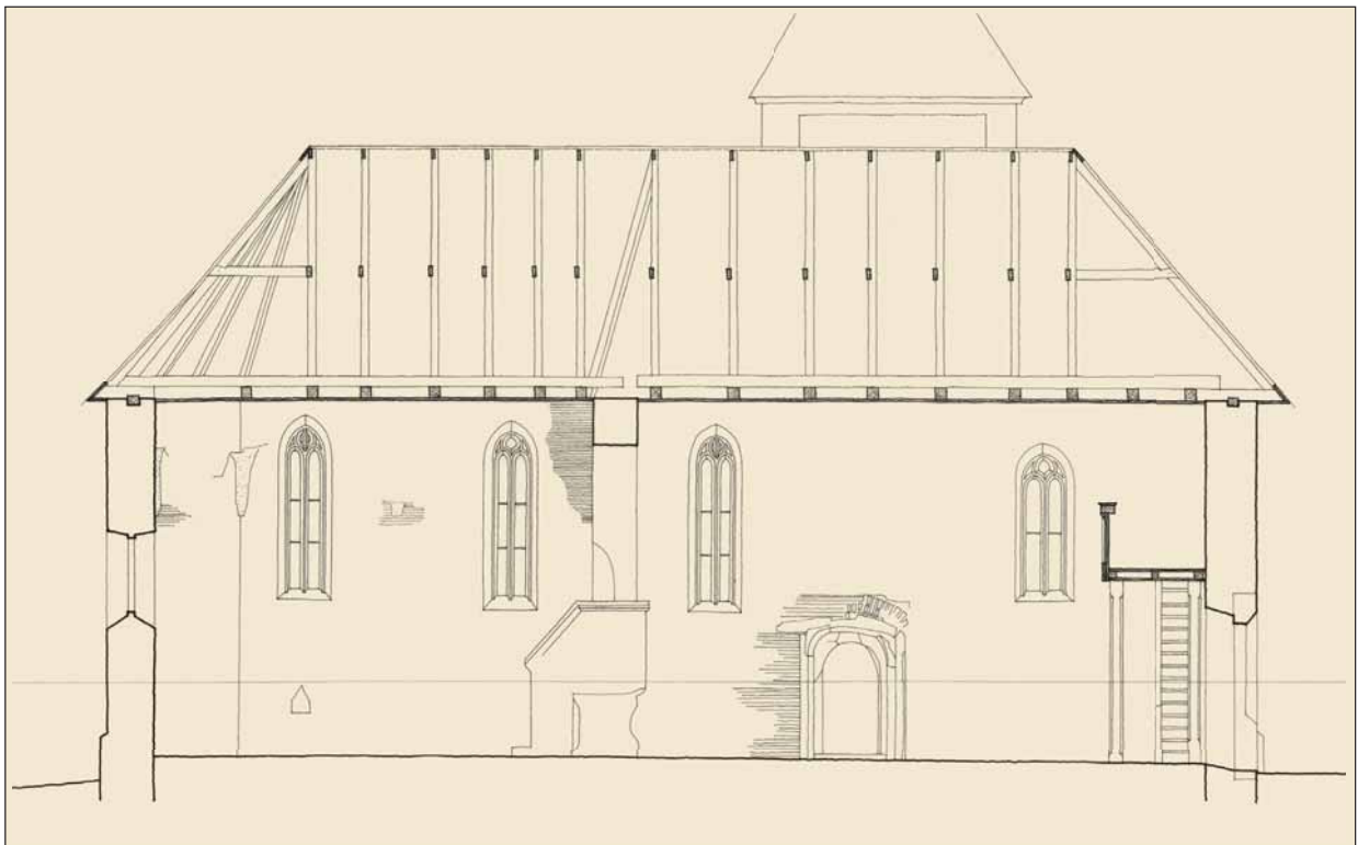
2. Secțiunea longitudinală a bisericii
